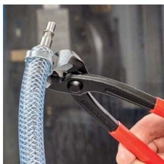
Étanher tuyau pneumatique au couplage rapide grâce au nez de pression frontal
