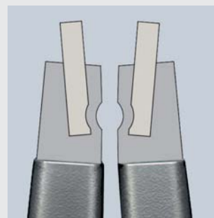
Pointes rapportées robustes en acier à ressort Sertissage précis par matriçage hautement comprimé
