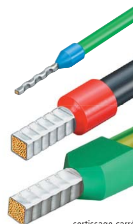
sertissage carré
